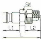
Műanyag tömlő-csatlakozó
