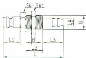
Szerelhető tömlőcsatlakozó
