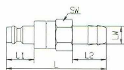
Tömítőcsatlakozó
