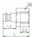
Belső menet
